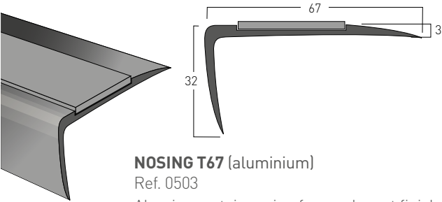
NOSING T67 (aluminium) Ref. 0503 Aluminum stair nosing for an elegant finish to steps while increasing safety with its non-slip strip. Nez de marche aluminium pour une harmonie palier/marche. Action anti-dérapante pour plus de sécurité.
