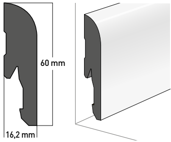
Ref. 5947 S001 MDF WHITE SKIRTING • Can be clipped (ref. 5948) • Nailed or adhesived • Can be painted over PLINTHE MDF BLANCHE • Peut être clipsée (réf. 5948) • Peut être clouée ou adhésivée • Peut être peinte
