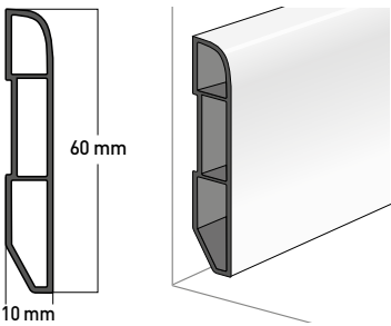
Ref. 6086 S001 VINYL WHITE SKIRTING • Water resistant • Can be adhesived • Can be painted over PLINTHE PVC BLANCHE • Résistante à l'eau • Peut être adhésivée • Peut être peinte
